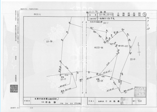
地積測量図
